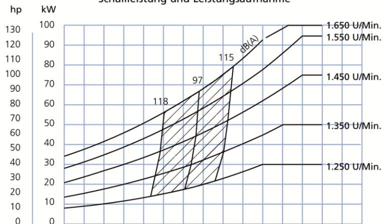
Schalleistung und Leistungsaufnahme
